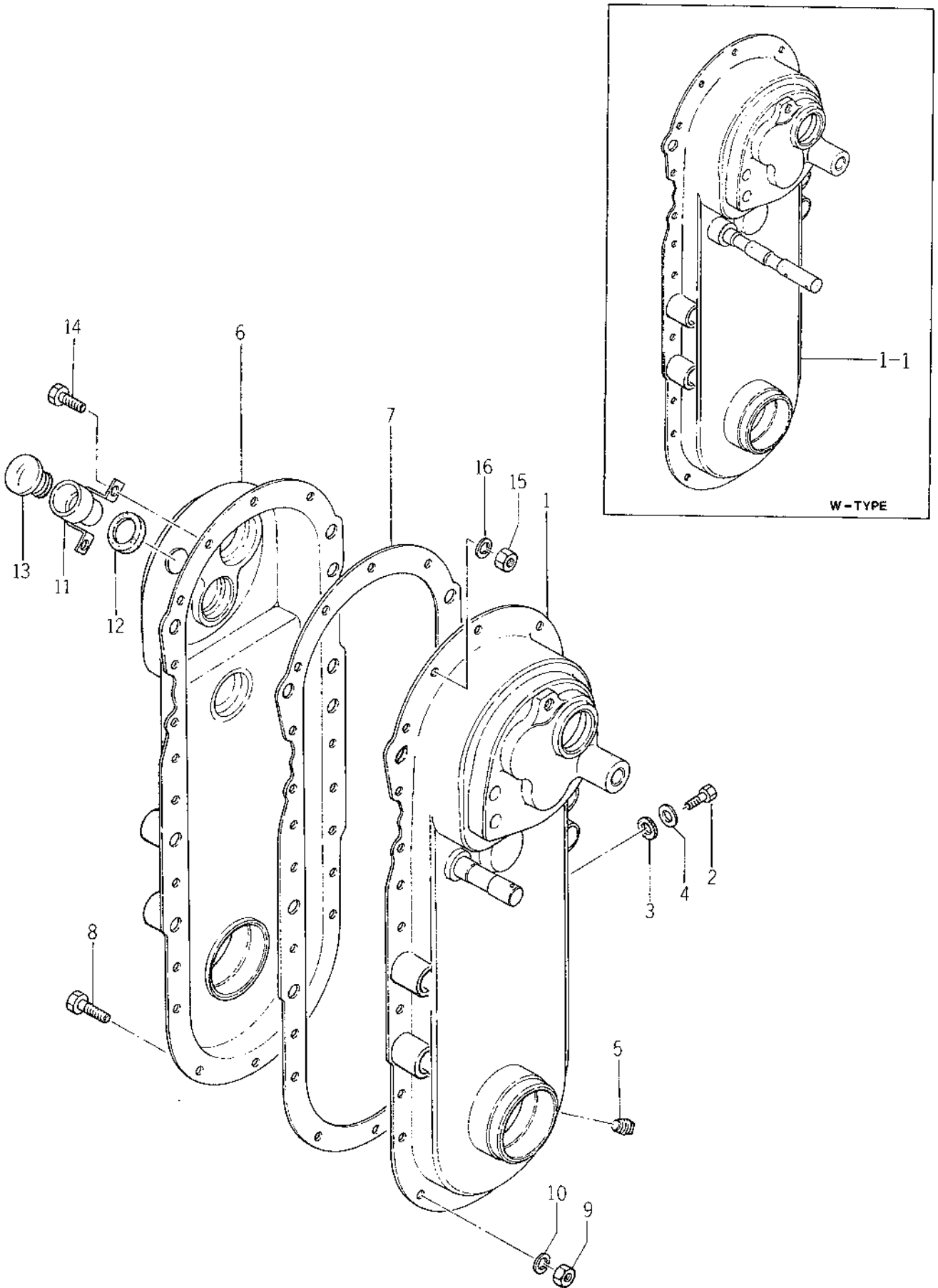
Fig. 7 TRANSMISSION GEAR CASE (For KC350) Boîtier de reducteur
