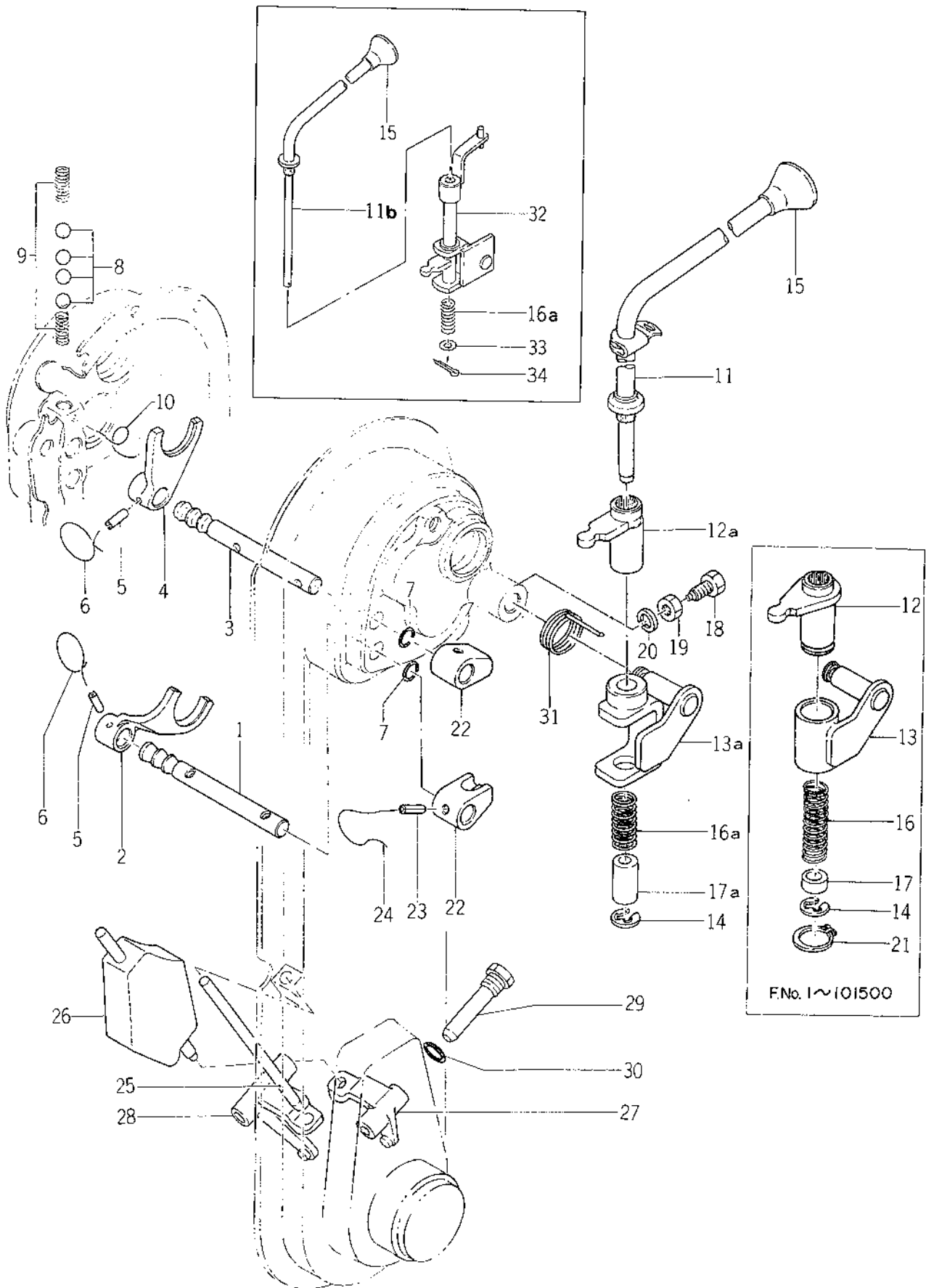
Fig. 10 SHIFTER Fourchettes
