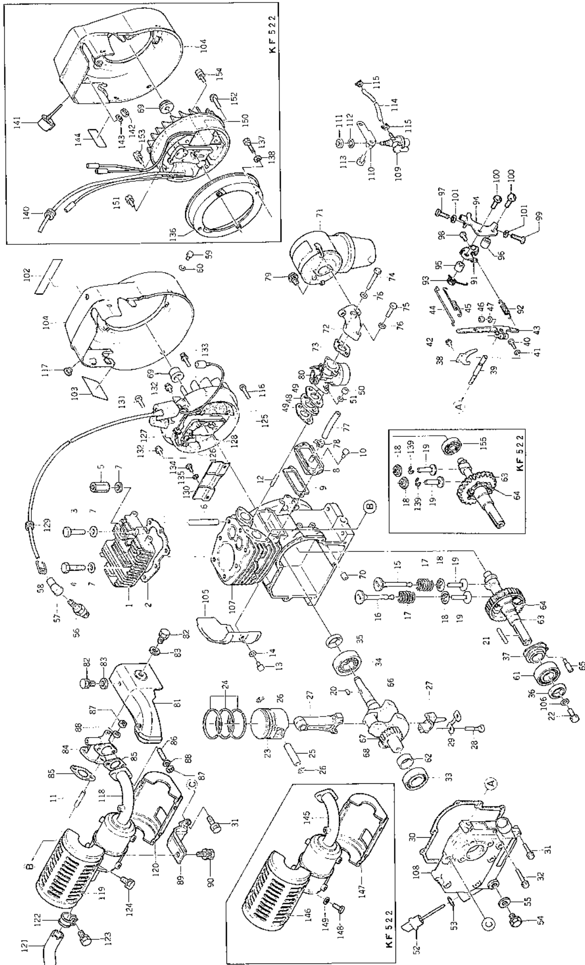
Fig. 1 ENGINE (KF522-A, KF522) Moteur (KF522-A, KF522)
