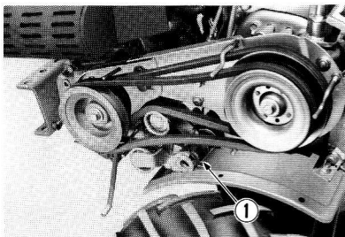
① Axe de bras de la poulie de tension
