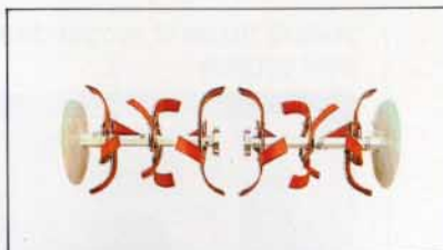
1. Rotors 'Labour' 6 étoiles et disques Ø 320mm largeur = 655mm Possibilité 2 étoiles additionnelles
