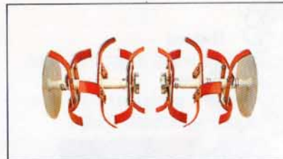
2. Rotors 'Standard' 6 étoiles et disques Ø 300mm largeur = 685mm Possibilité 2 étoiles additionnelles
