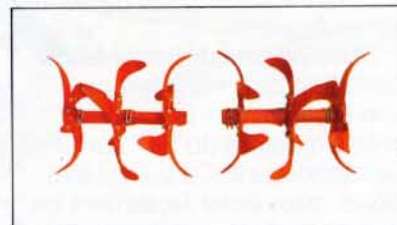
3. Rotors 'Hélice' 6 étoiles Ø 310mm largeur = 765mm Possibilité 2 étoiles additionnelles
