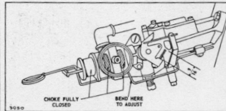
Fig. 65 - Choke Idle Return
