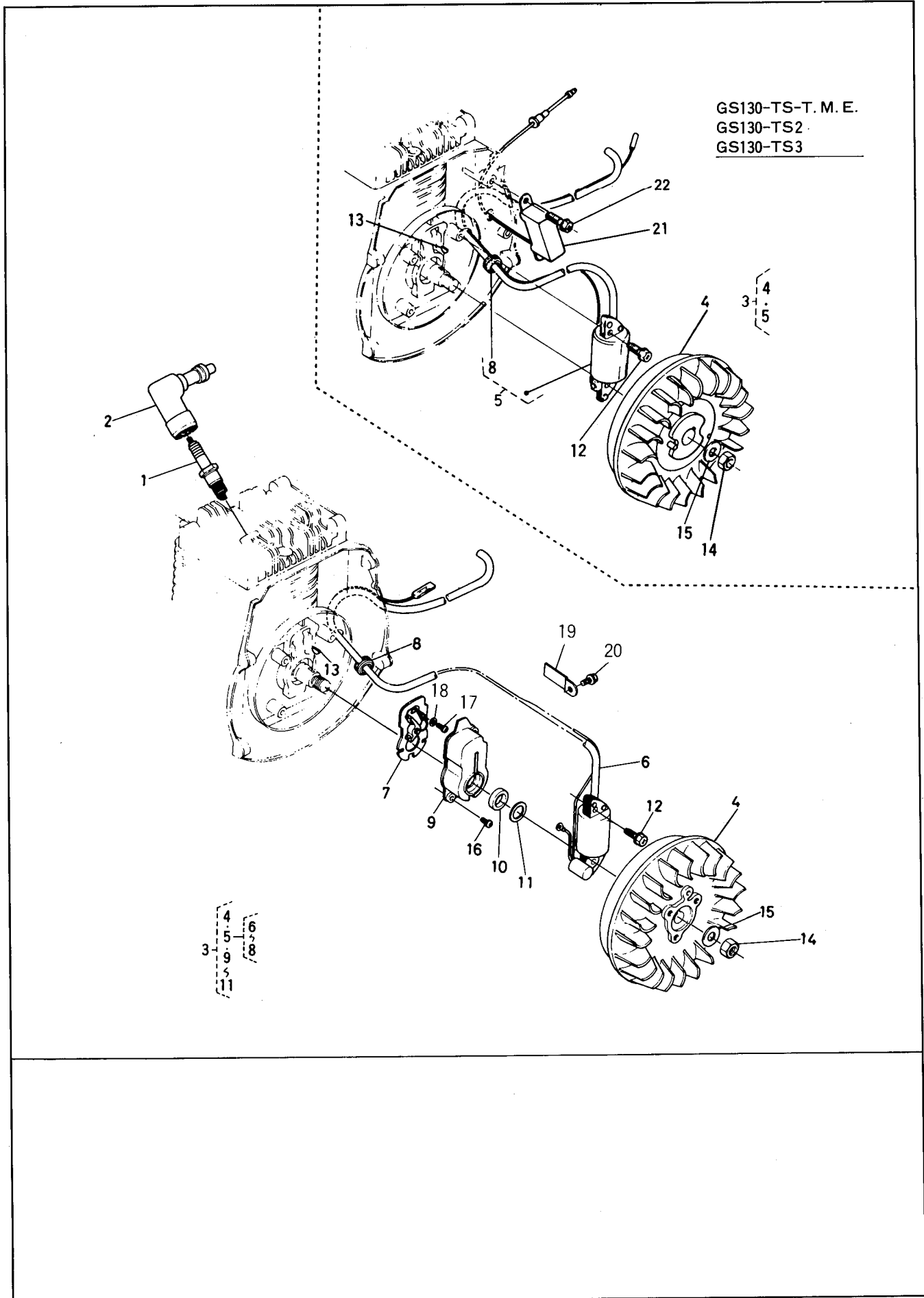
FIG. 10 VOLANT MAGNETIQUE MAGNETO MAGNETZÜNDER
