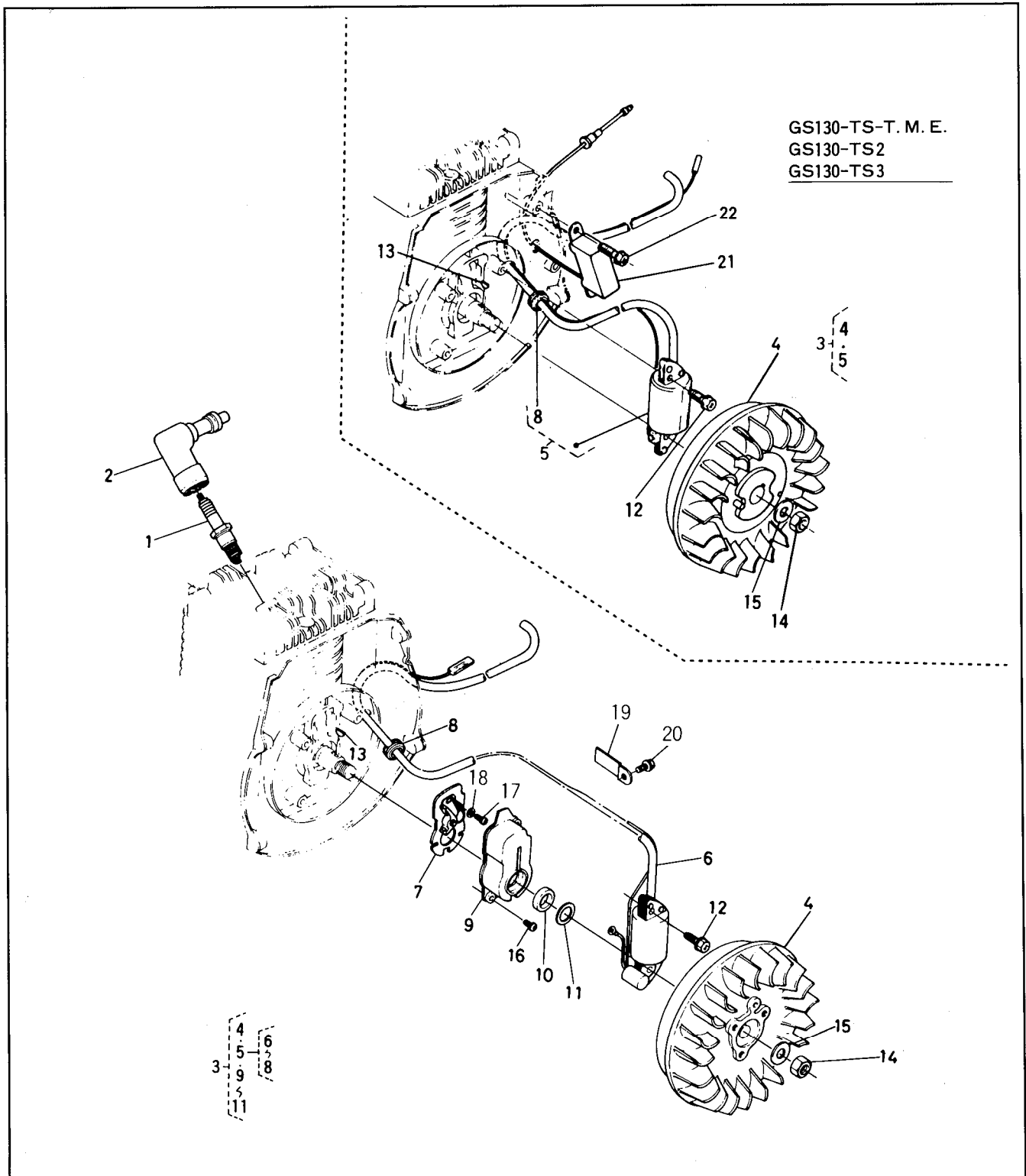
FIG. 10 VOLANT MAGNETIQUE MAGNETO MAGNETZÜNDER
