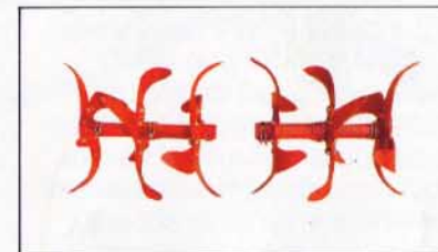
3. Rotors 'Hélice' 6 étoiles Ø 380mm largeur = 1.075mm Possibilité 2 étoiles additionnelles
