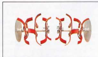
2. Rotors 'Standard' 6 étoiles et disques Ø 360mm, largeur = 1.020mm Possibilité 2 étoiles additionnelles
