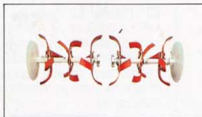
1. Rotors 'Labour' 6 étoiles et disques Ø 360mm largeur = 875mm Possibilité 2 étoiles additionnelles
