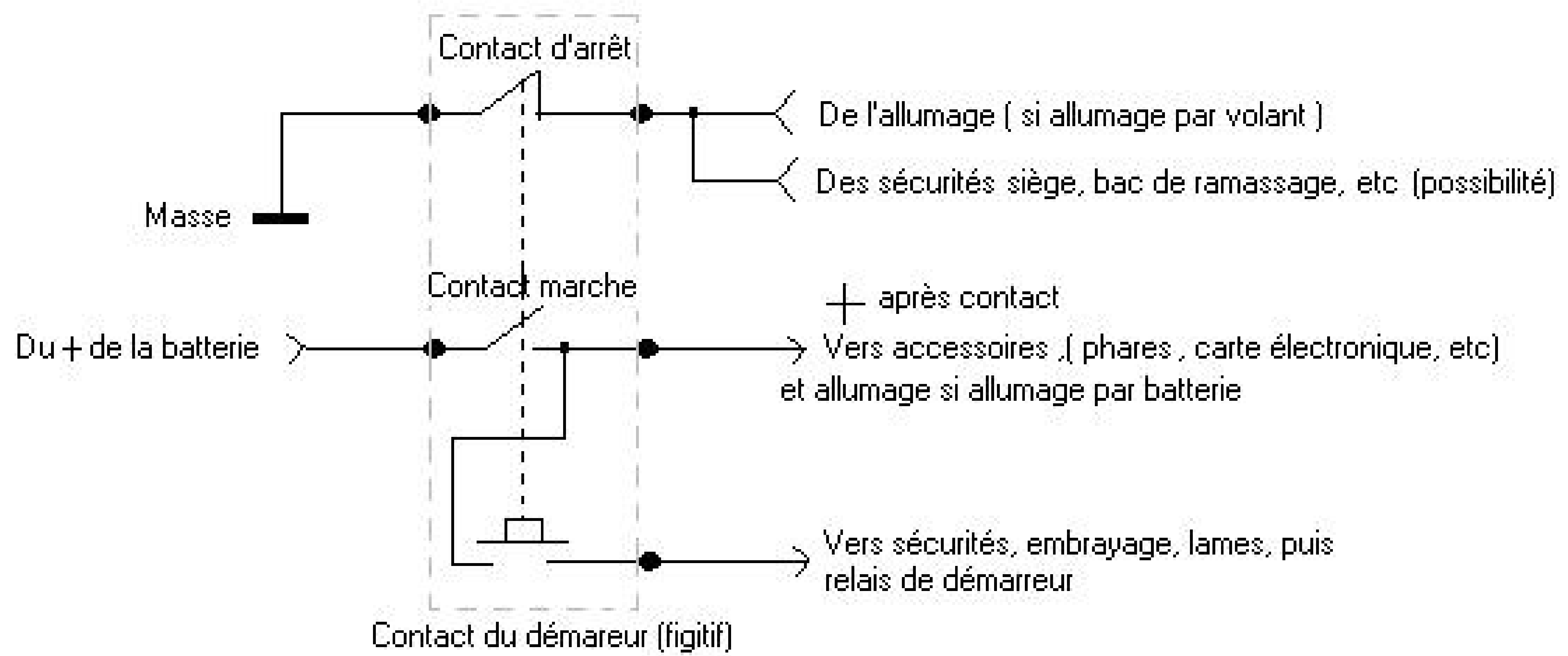
Contacteur représenté en position arrêt
