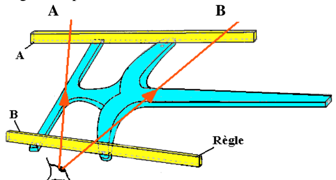
Contrôle du parallélisme de l'âge et étançons
