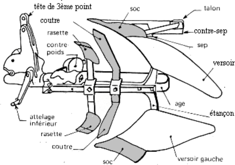
Charrue brabant demi tour pour microtracteur
