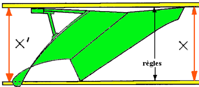
Contrôle de la capacité ou largeur de travail
