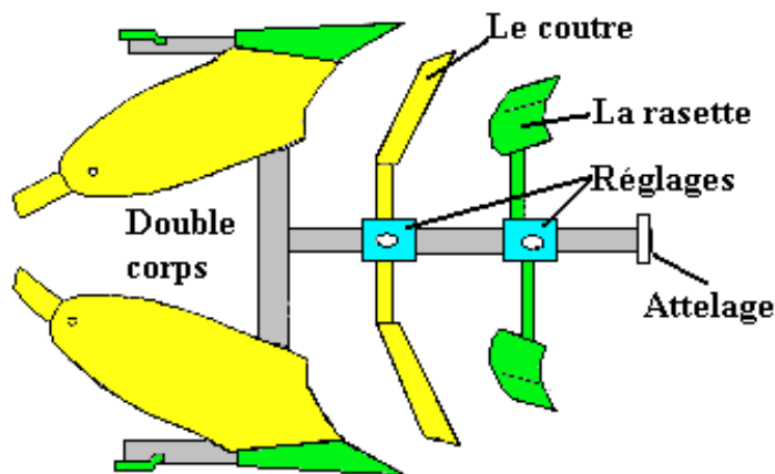
Représentation d'une charrue brabant demi-tour
