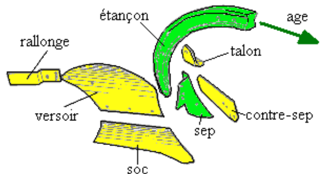
Eclaté d'un corps de charrue classique
