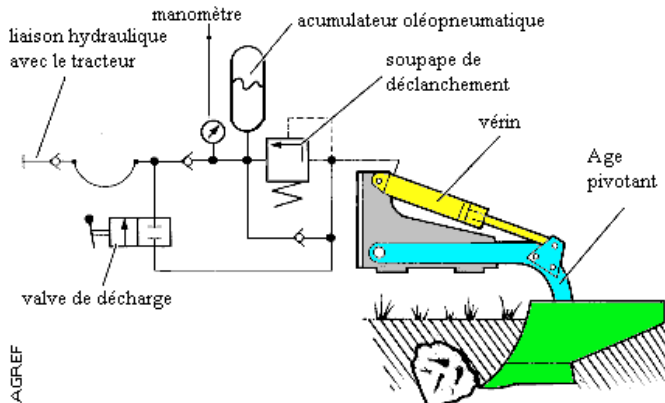
Charrue agricole avec système de sécurité non stop hydraulique
