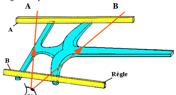
Contrôle du parallélisme de l'âge et étauçons
