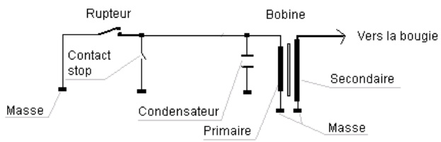
Allumage à rupteur par volant magnétique
