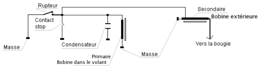
Allumage à rupteur par volant magnétique à bobines séparées
