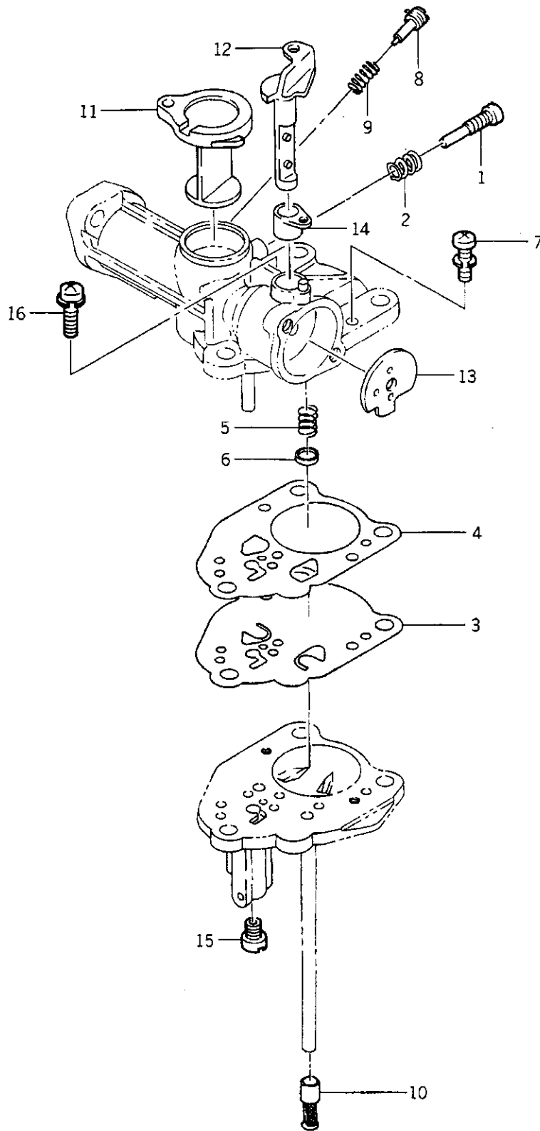
Fig. C-1 CARBURETOR
