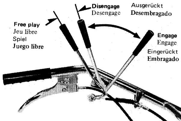
Main clutch adjuster Lévier de réglage d'embrayage principal Hauptkupplungs-Einstellschraube Ajustador de embrague principal
