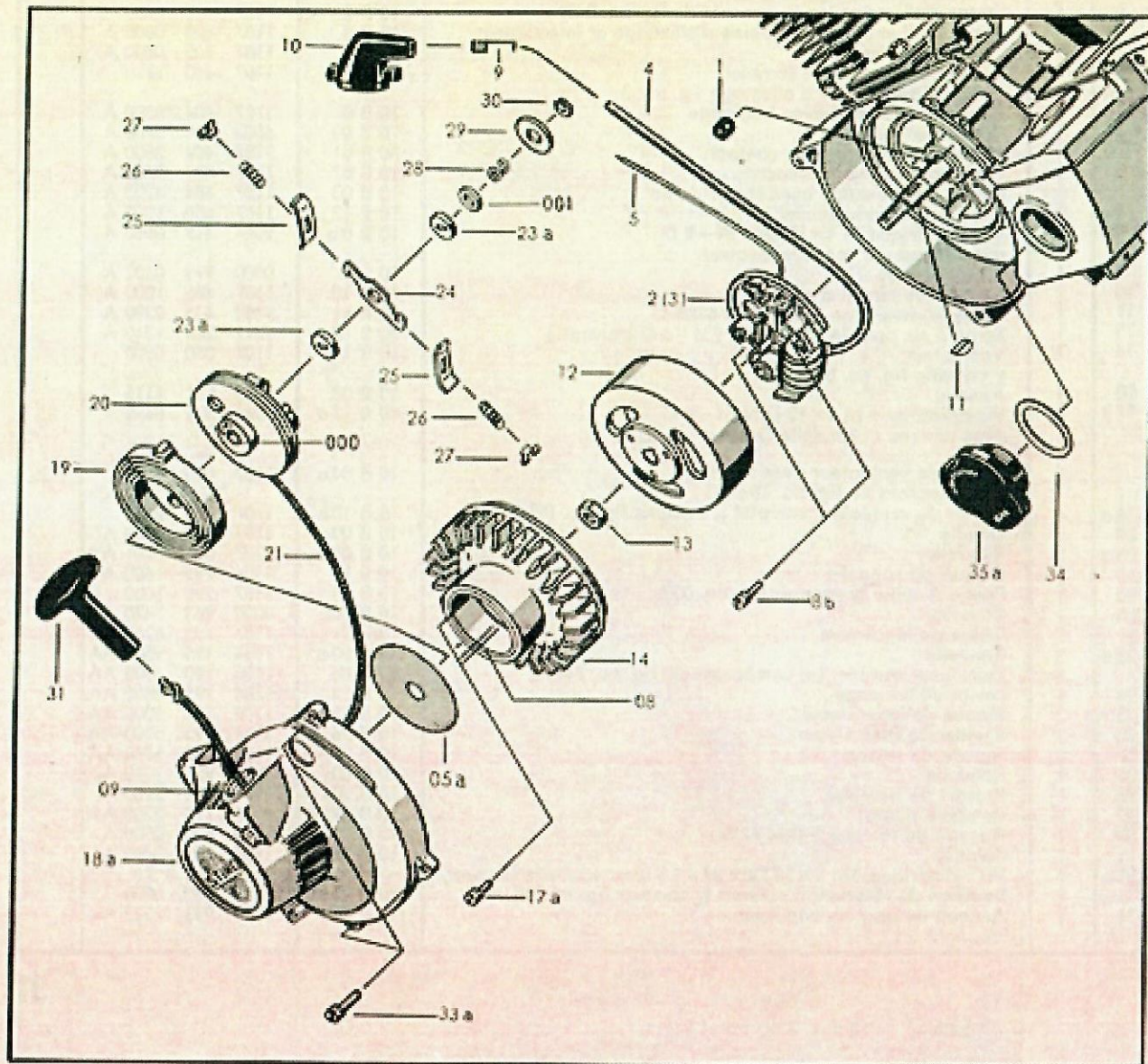
Illustration B Volant magnétique, Ventilateur, Carter de ventilateur, Lanceur
