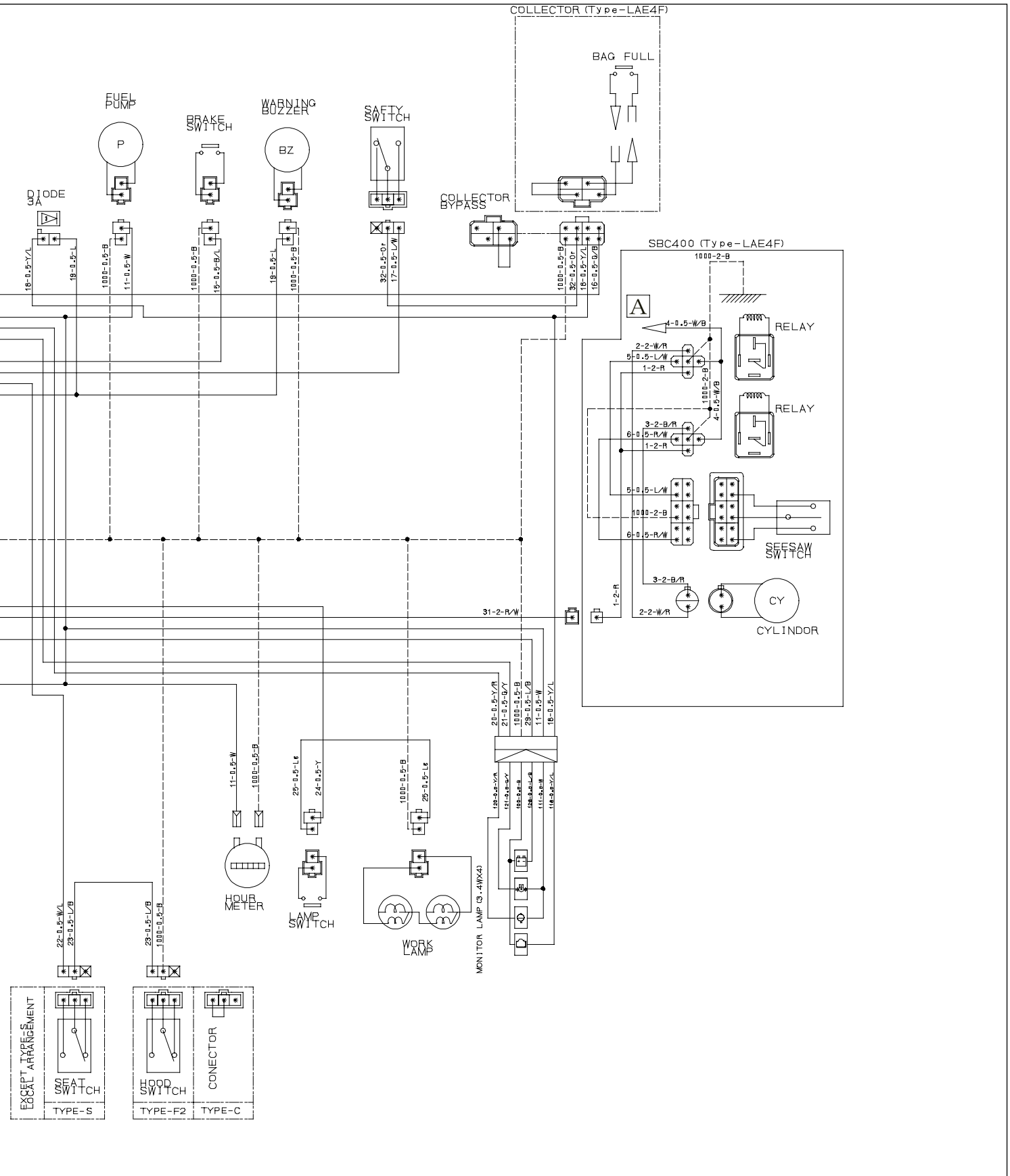
VERKABELUNGSDIAGRAMM
